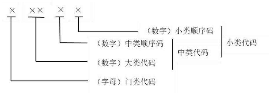
图 1 代码结构图
